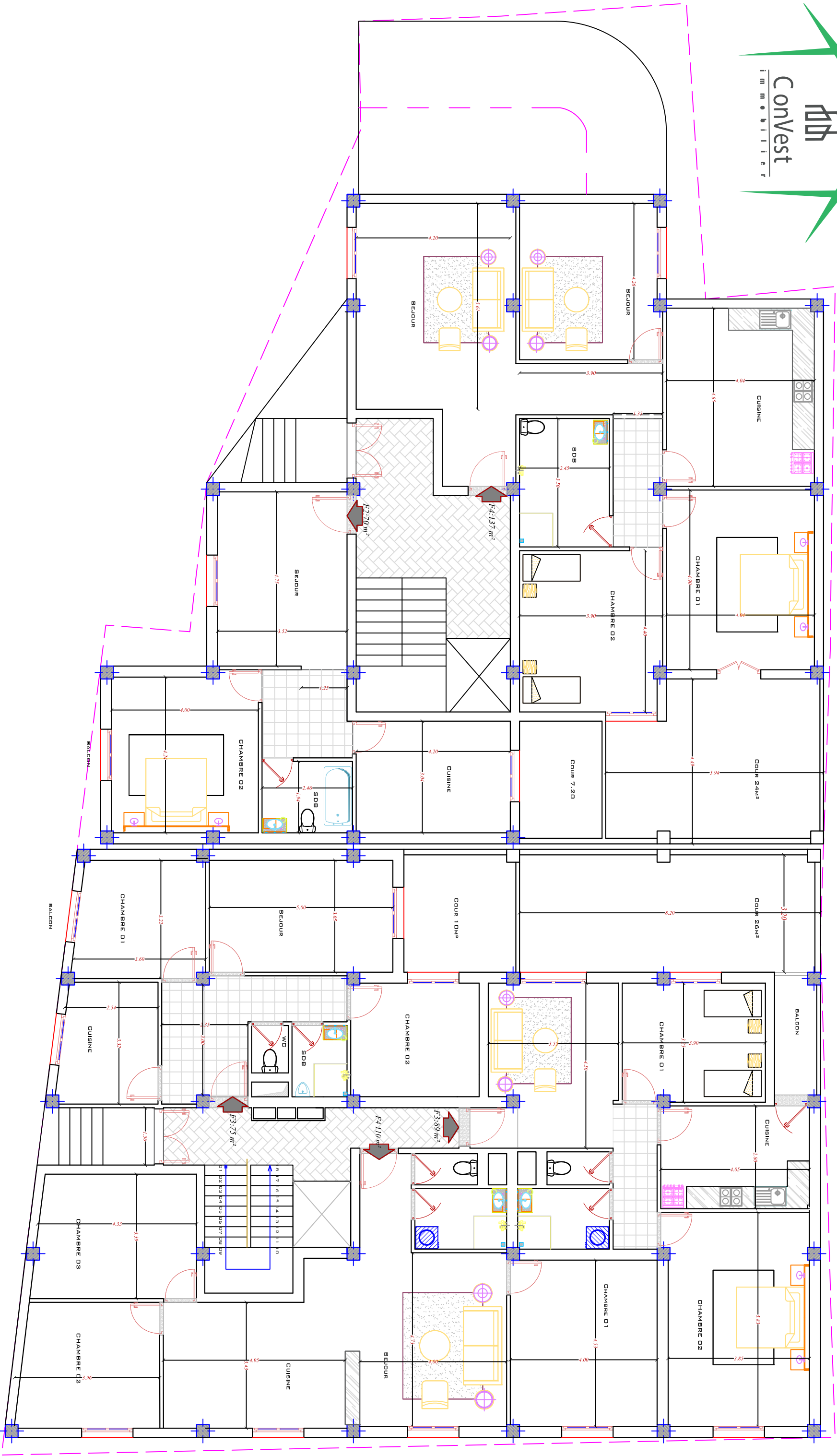
PLAN RDC
